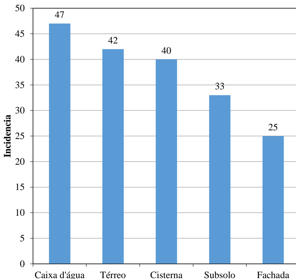
Figura 5. Localização das manifestações patológicas. Caixa d'água; Térreo; Cisterna; Subsolo; Fachada
