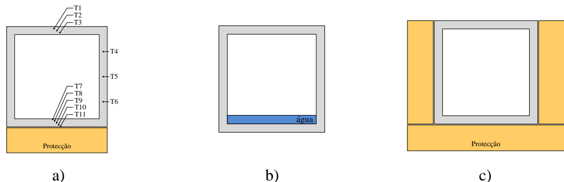
Figura 1. (a) Vigas con protección pasiva expuestas a una cara (siendo indicada la posición de las termocuplas); (b) vigas con protección activa expuestas a un tercio de cara(s); e (c) viga con protección pasiva expuesta en las tres caras.
