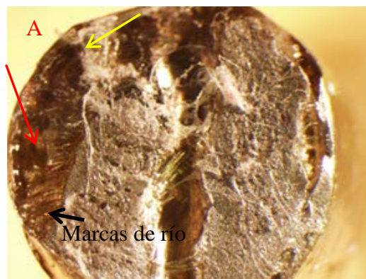
Figura 11A. Fratura da amostra com bisel individual com terceiro Inconel. Observa-se falta de fusão (seta vermelha) e cavidades (seta amarela) na fratura.
